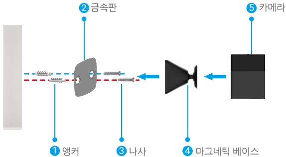
그림 2. 나사로 장착
